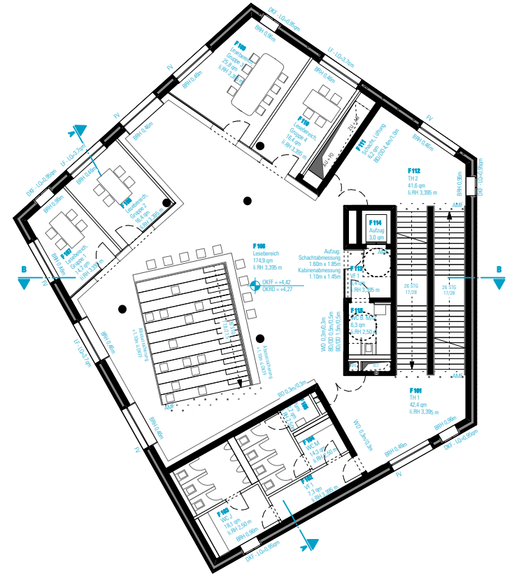
1. Obergeschoss
